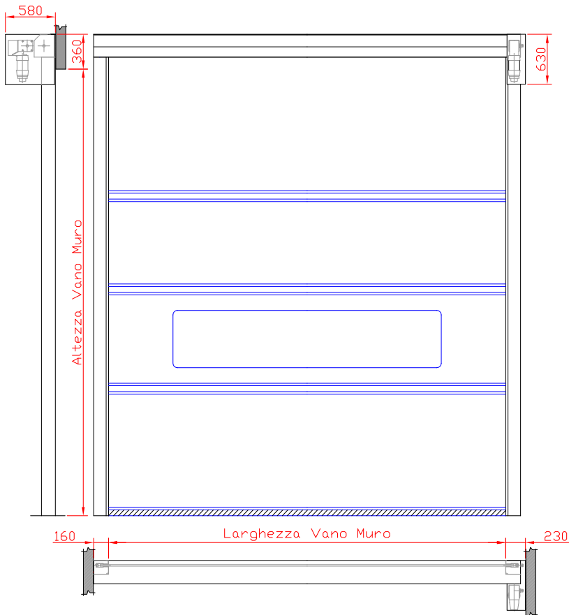
Motore laterale
