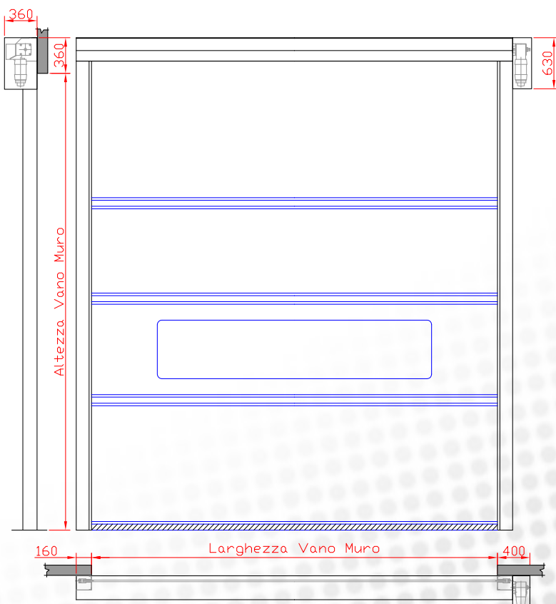
Motore laterale
